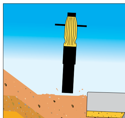
Figur 3.56. Komprimering af stabilt grus bag trinnet eventuelt ved brug af brolæggerjomfru.
