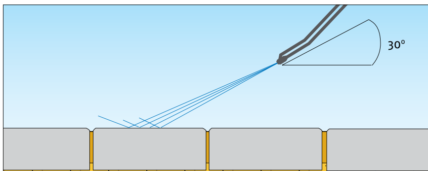
Figur 4.4. Hvis der anvendes højtryksrensere skal strålens vinkel med vandret maks. være 30^\circ .
